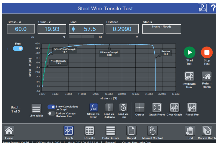
Visualisation d'une courbe de contrainte-déformation avec les calculs annotés sur les tests de matériaux.
